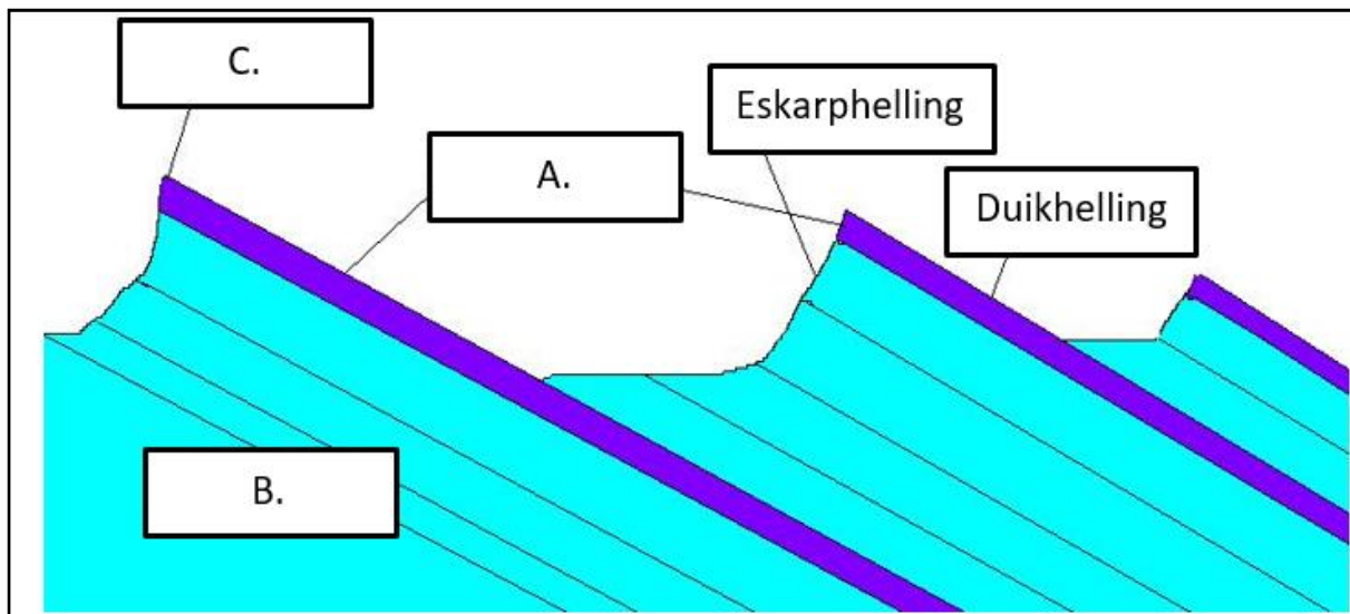
FIGUUR 2.6 HELLENDE LAE
